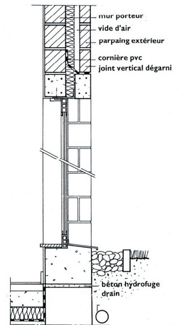
coupe de détail sur mur double
